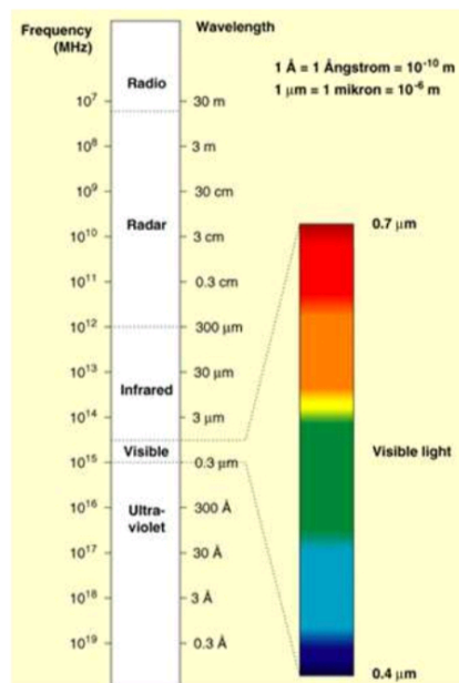
1.4: विद्युत चुम्बकीय स्पेक्ट्रम (a) प्रमुख प्रभाग (b) उनकी तरंग दैर्घ्य और आवृत्तियों के साथ विभाजन।
