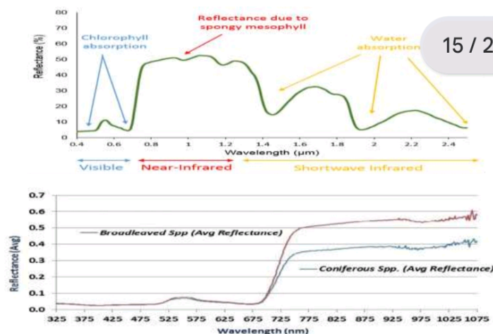
चित्र 1.6: वनस्पति का वर्णक्रमीय हस्ताक्षर दर्शाता है: क) स्वस्थ वनस्पतियों और बी) शंकुधारी और चौड़ी पत्ती वाली प्रजातियों के बीच अंतर। क्लोरोफिल की मात्रा अधिक होने के कारण शंकुधारी प्रजातियों की तुलना में चौड़ी पत्ती वाली प्रजातियाँ एनआईआर क्षेत्र में अधिक परावर्तन दिखाती हैं।
